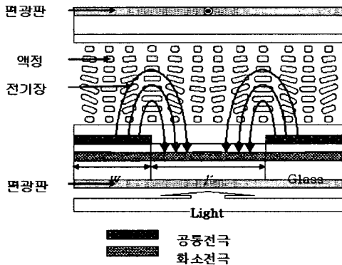
그림 1. 옆에서 본 FFS의 밝음 상태에서 액정 방향자.
