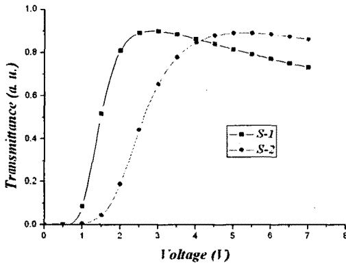
그림 4. 전압인가에 따른 투과율 곡선.
