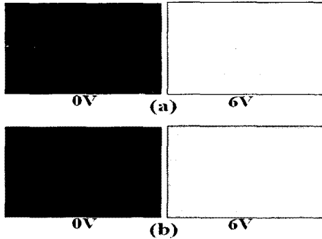
그림 6. (a)C-1과 (b)C-2에 각각 0V와 6V 를 인가 한 후의 현미경사진.
