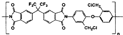
그림 2. 클로로메틸레이티드 폴리이미드 (CMPI) 고분자 구조.
