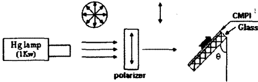
그림 3. 사용된 UV 조사 장치.
