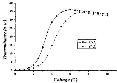
그림 5. 전압인가에 따른 투과율 곡선.
