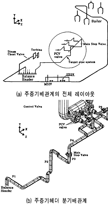
Fig. 1. 발전소 주증기배관계 및 대상 분기배관계의 레이아웃
