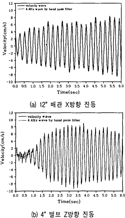
Fig. 2. 주증기 분기 배관계의 집중질량부 진동 파형
