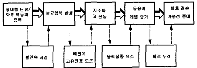
Fig. 5. 배관계의 진동 건전성 평가 절차
