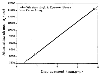
(a) 진동 변위와 동응력
