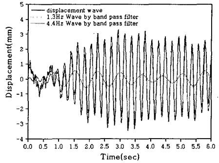
(a) 대책전 4°배관 Z방향의 진동
