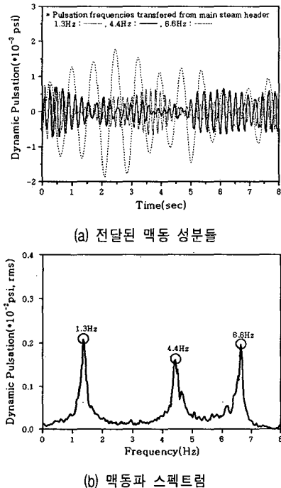
Fig. 3. 분기 배관계에 전달된 광대역 난류 맥동파 특성
