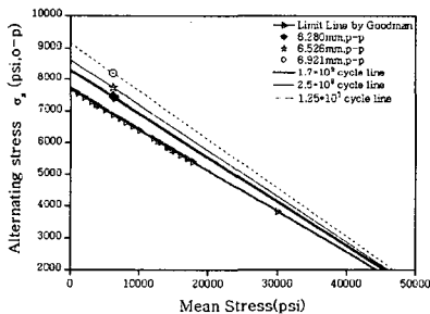
(b) 4"배관의 피로응력
