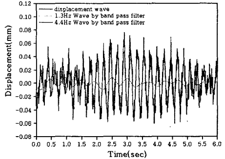
(b) 대책후 4°배관 X방향의 진동
