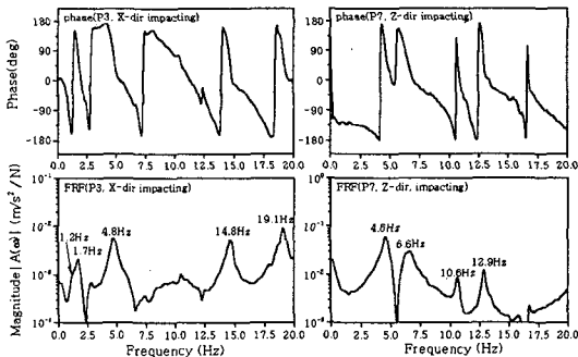
(b) 고유진동수 응답함수
