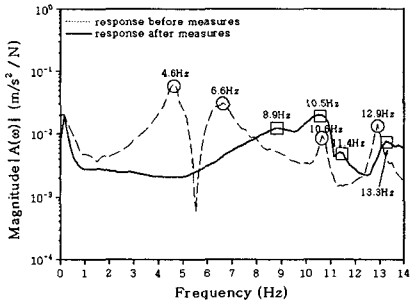
(b) 피로누적상태의 4°배관계의 응답
