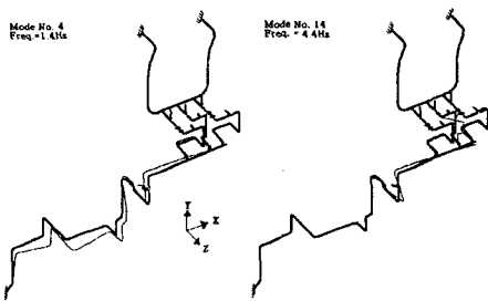
(a) 배관계의 주요 고유진동 모드
