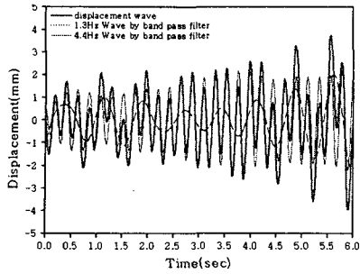
(a) 12" 배관의 변위 파형
