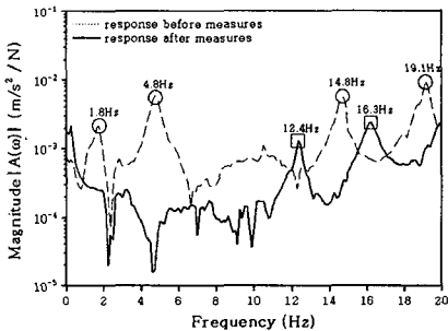
(a) 정지밸브가 설치된 12°배관의 응답
