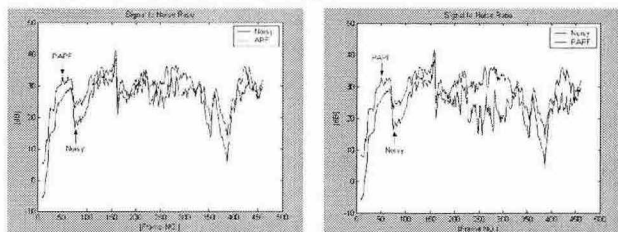
(a) APF의 SSNR (b) PAPF의 SSNR
