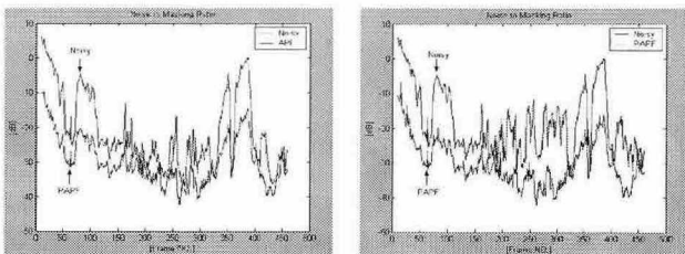
(a) APF의 NMR (b) PAPF의 NMR
