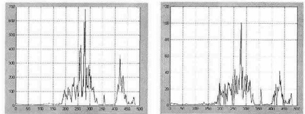
(a) APF의 연산량 (b) PAPF의 연산량 그림 1. 30dB 에서 APF, PAPF의 연산량 비교
