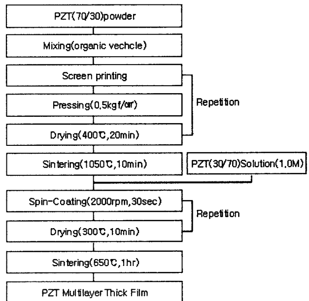
〈그림 1〉 PZT 후막의 제작공정.
