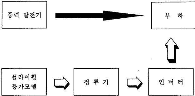
〈그림 4〉 전력안정화시스템 Blockdiagram
