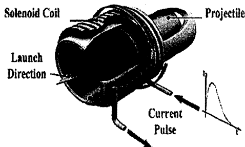
<그림 2> 솔레노이드형 EML의 구조와 원리
