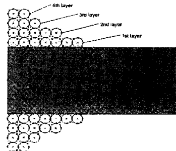
<그림 3> 솔레노이드의 코일 적층 형태
