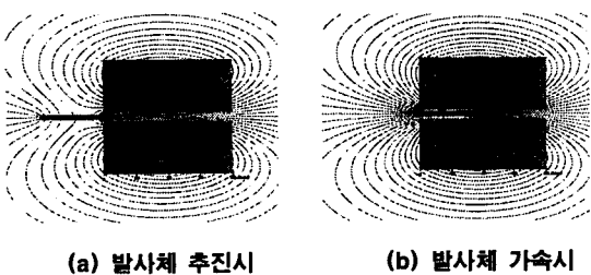
〈그림 5〉 발사체가 추진, 가속할 때의 자속밀도 분포
