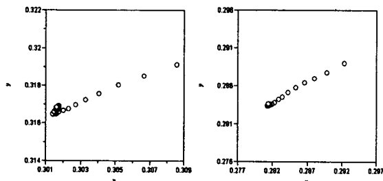
〈그림 4〉 시간에 따른 LED Module 색좌표 특성
