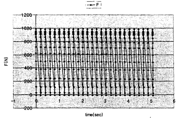
〈그림 4〉 시간변화에 따른 전자력
