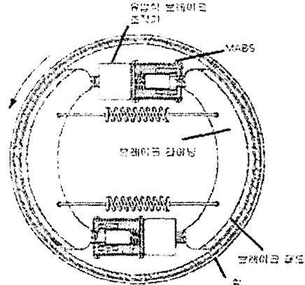
<그림 1> 휠 브레이크 내부 구조
