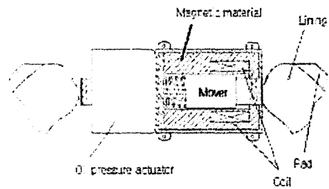
<그림 2> MABS와 유압조작기 세부구조
