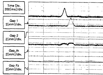
〈그림 10〉 공극입력신호 및 스텝시홀드에 의한 공극과 퍼지에 의한 공극(단차 없음)
