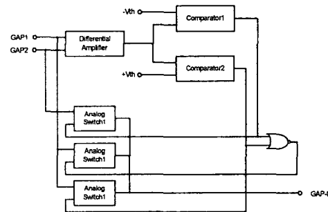
〈그림 3〉 듀얼 공극신호 처리 개념도
