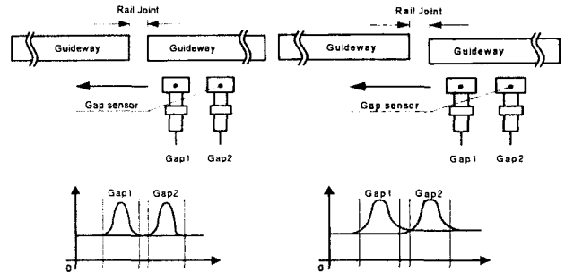
〈그림 1〉 주행시 공극신호 (단차 없는 경우)
