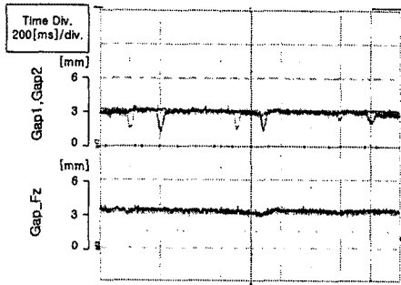
〈그림 11〉 주행시 퍼지에 의한 공극제어
