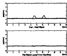
〈그림 6〉 공극 및 퍼지에 의한 공극 (저속주행, 단차없음)
