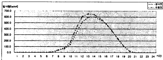
(c) 수평면 일사량과 경사면 일사량
