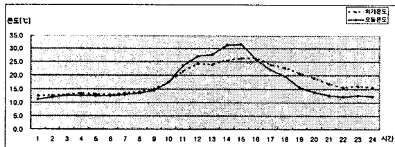
(b) 외기 온도와 태양전지 모듈온도
