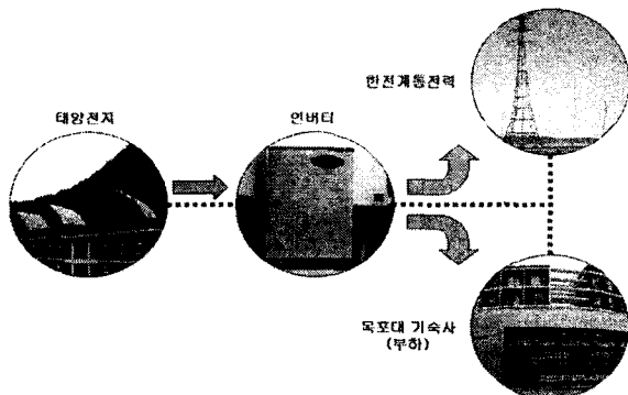
<그림 1> 30kW 계통연계형 태양광발전시스템 전체구성도
