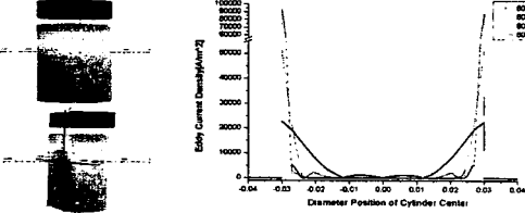
〈그림 6〉 1번 모델의 와전류 분포 및 와전류 패턴
