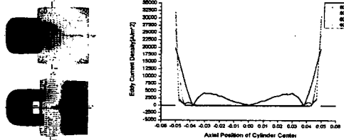
〈그림 5〉 1번 모델의 와전류 분포 및 와전류 패턴
