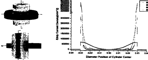
〈그림 4〉 4번 모델의 와전류 분포 및 와전류 패턴
