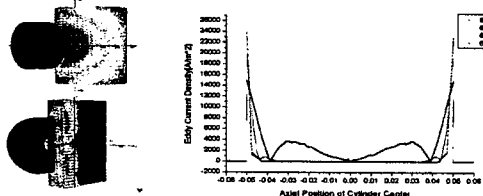
〈그림 2〉 2번 모델의 와전류 분포 및 와전류 패턴
