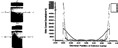
〈그림 3〉 3번 모델의 와전류 분포 및 와전류 패턴
