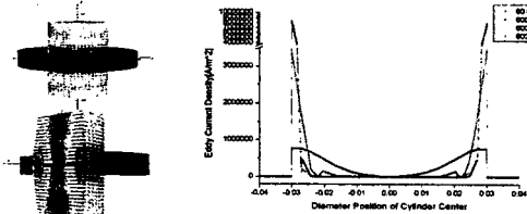
〈그림 1〉 1번 모델의 와전류 분포 및 와전류 패턴
