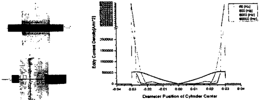
〈그림 7〉 1번 모델의 와전류 분포 및 와전류 패턴
