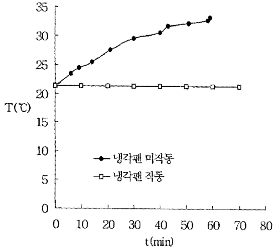
Fig. 3 히트파이프의 응축부의 온도변화
