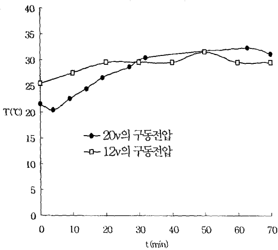
Fig. 7 히트파이프 및 냉각팬이 설치된 구동모터의 전압차이에 의한 온도변화 (Fig. 2 ②)
