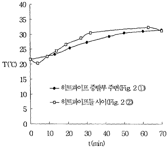
Fig. 6 열전대의 측정위치 변화에 따른 온도 변화
