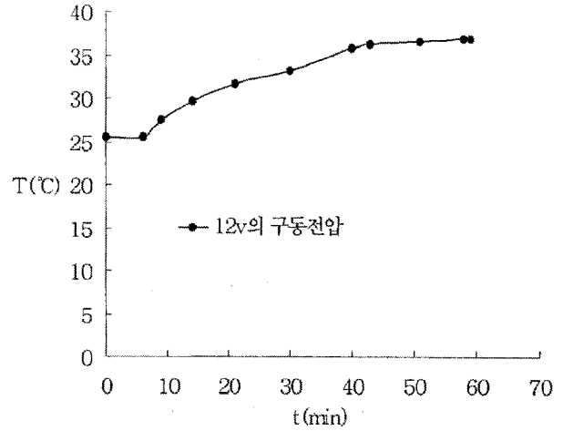
Fig. 5 히트파이프에 의한 구동모터의 온도변화 (Fig. 2 ㉔)
