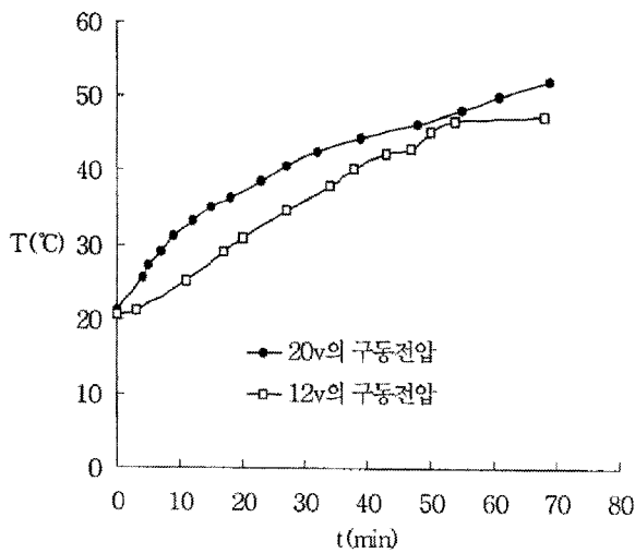
Fig. 4 전압차이에 의한 구동모터의 온도변화 (Fig. 2 ㉔)
