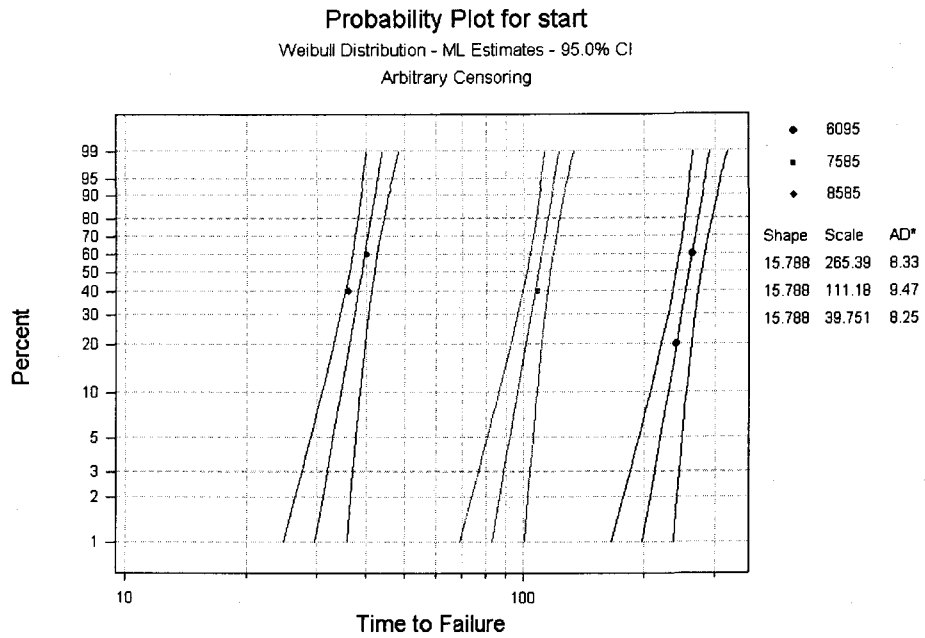
그림 3. 와이블 확률지 타점 결과
