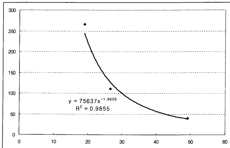
그림 4. 와이블분포의 척도모수와 수증기압 사이의 관계
