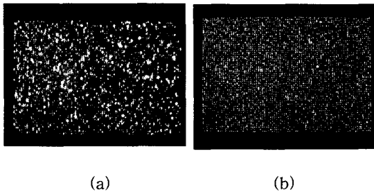
Fig. 4. The field emission image of (a) before and (b) after aging of herringbone CNF emitters 그림 4. 에이징 공정에 따른 발광이미지 변화 (a) 에이징 전 및 (b) 에이징 후
