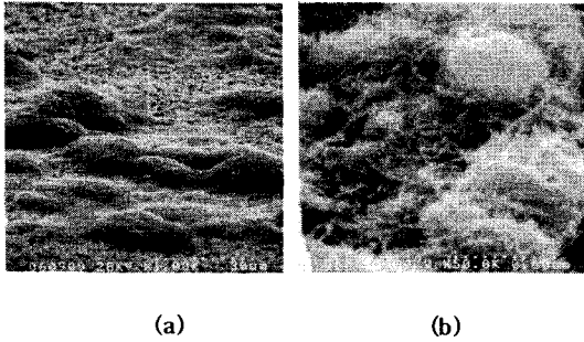
Fig. 2. SEM image of (a) as screen-printed and after surface-treatment of herring-bone types CNF 그림 2. CNF 해링본-구조의 표면처리 사진 (a) 표면처리 전 및 (b) 표면처리 후
