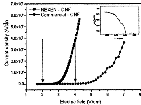
Fig. 3. I-V and Fowler-Nordheim plot of herringbone CNF in screen-printing process 그림 3. 인쇄방식으로 제조된 해링본 구조 CNF의 전류 및 전압 변화
