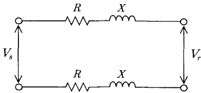
(그림 2) 교류 단상2선식 등가회로
