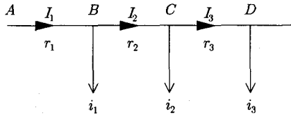
(그림 3) 직류2선식 분산부하 배선도
