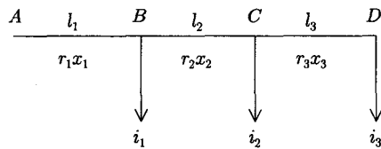
(그림 4) 교류 단상2선식 분산부하 배선도
