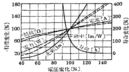
(그림 1) 전구의 전압변화에 의한 특성, 수명변화
