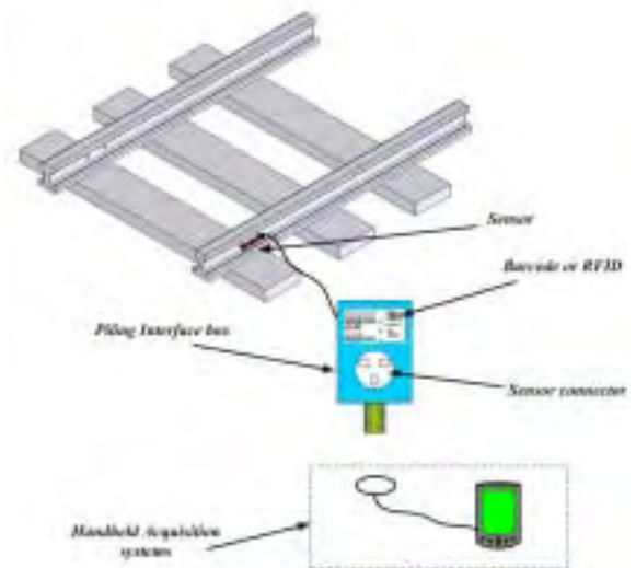
그림 4 장대레일 축응력 계측 시스템
