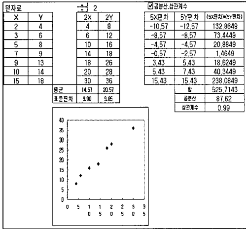
[그림 7] 원자료를 2배 증가했을 때의 공분산과 상관계수
