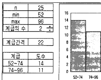
[그림 4] 계급의 수가 2일 때 히스토그램
