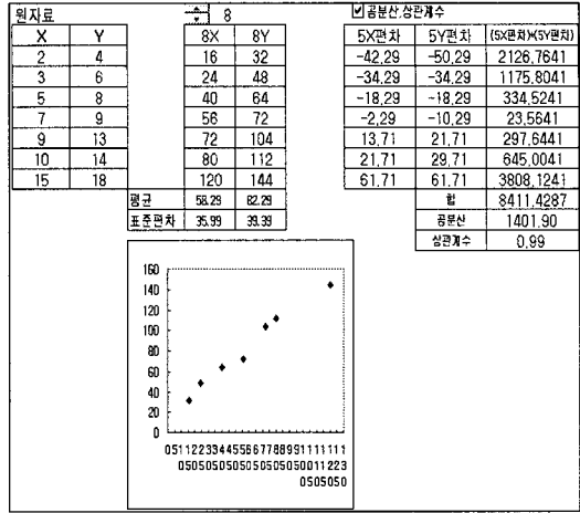
[그림 8] 원자료를 8배 증가했을 때의 공분산과 상관계수
