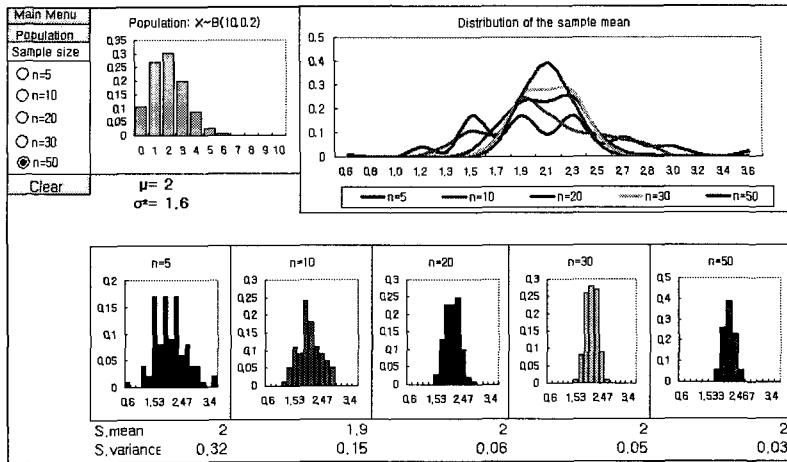
[그림 14] 중심극한정리
