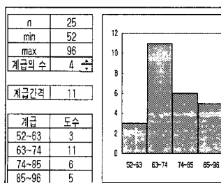
[그림 5] 계급의 수가 4일 때 히스토그램
