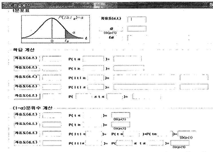
[그림 13] t분포 확률계산
