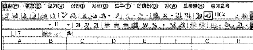
[그림 1] 초기화면
