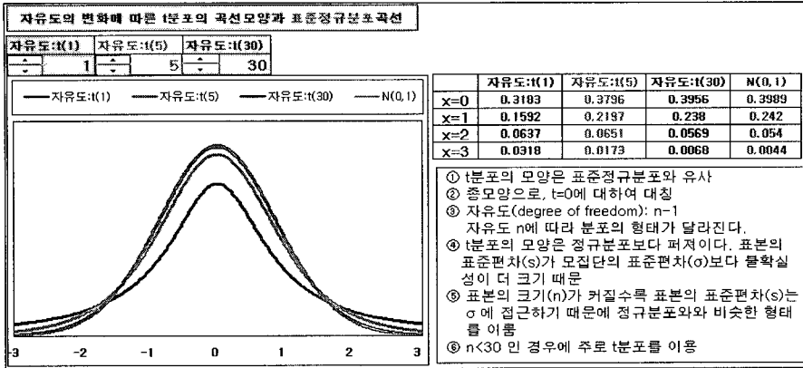
[그림 12] 자유도 변화에 따른 t분포 곡선과 표준정규분포곡선
