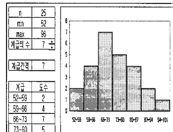
[그림 6] 계급의 수가 7일 때 히스토그램
