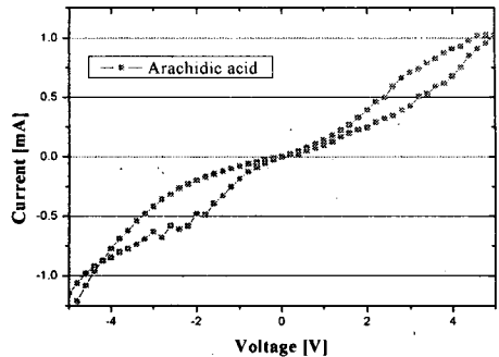
그림 3. Arachidic acid의 I-V특성 곡선
