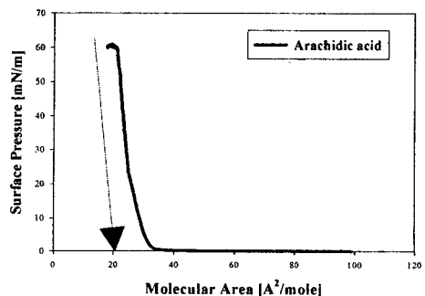
그림 1. Arachidic acid의 \pi -A 등온선
