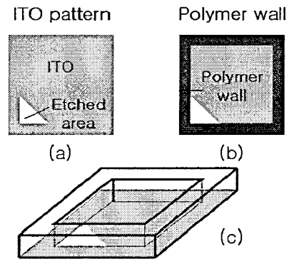
그림 1. 하부 기판의 전극 패턴과 고분자 벽의 형성
