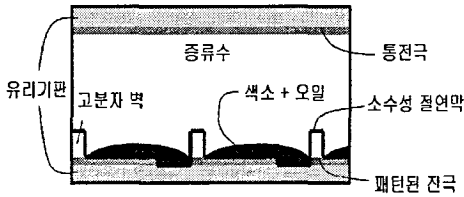
그림 2. Electrowetting display 테스트 셀 구조도
