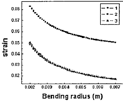
그림 2. Strain of Type1, Type2, Type3.
