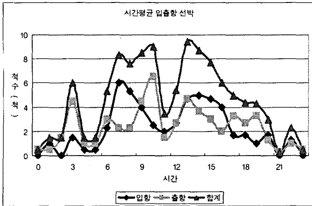
<그림 11> 시간평균 입항 및 출항선박분포
