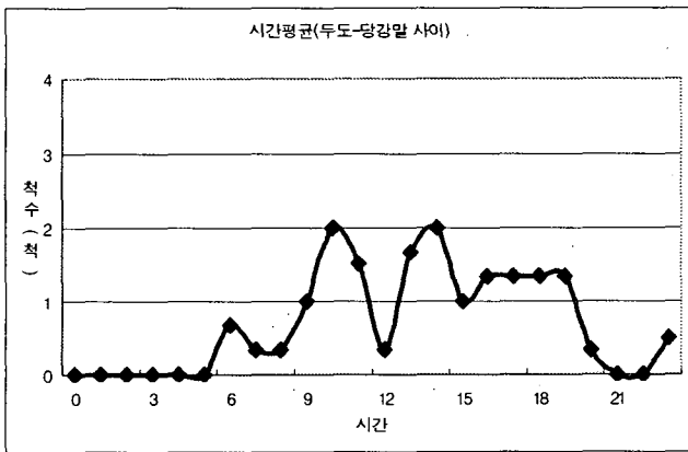
<그림 18> 두도-당강말 사이의 전일시간평균 횡단선박
