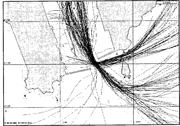
<그림 7> 입항 선박의 항적
