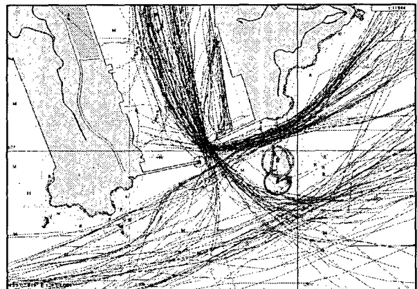
<그림 4> 어선의 항적
