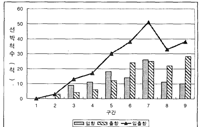
<그림 24> 각 횡단구간별 통과선박
