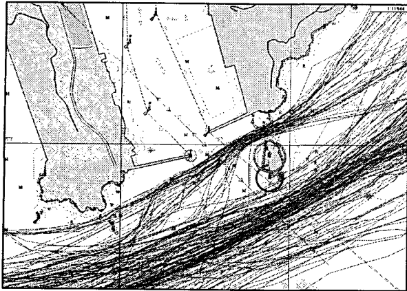
<그림 9> 외항항로의 횡단선박항적
