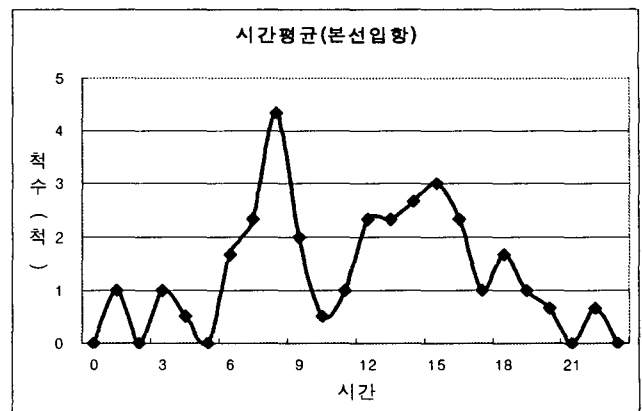
<그림 13> 지정항로 이용 전일시간평균 입항선박
