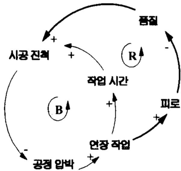
그림 1. 인과관계루프 다이어그램 예
