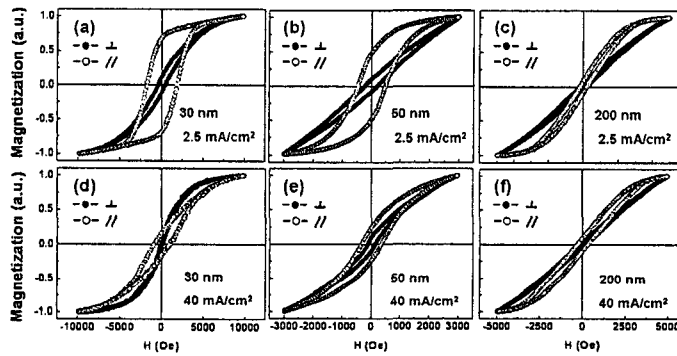
Fig. 1. 전류밀도에 따른 나노 템플레이트에 전착된 지름 200nm, 50nm, 30nm Co 나노선의 hysteresis loop
