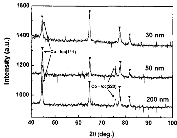
Fig. 2. 나노 템플레이트에 전착된 지름 200nm, 50nm, 30nm Co 나노선의 XRD 분석결과
