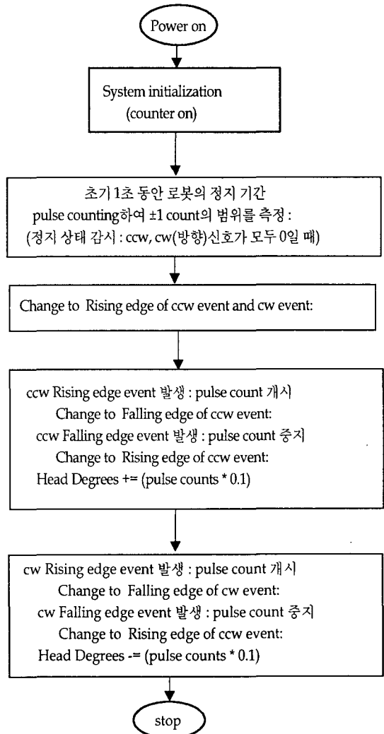
그림 4. 각속도 측정을 위한 흐름도
