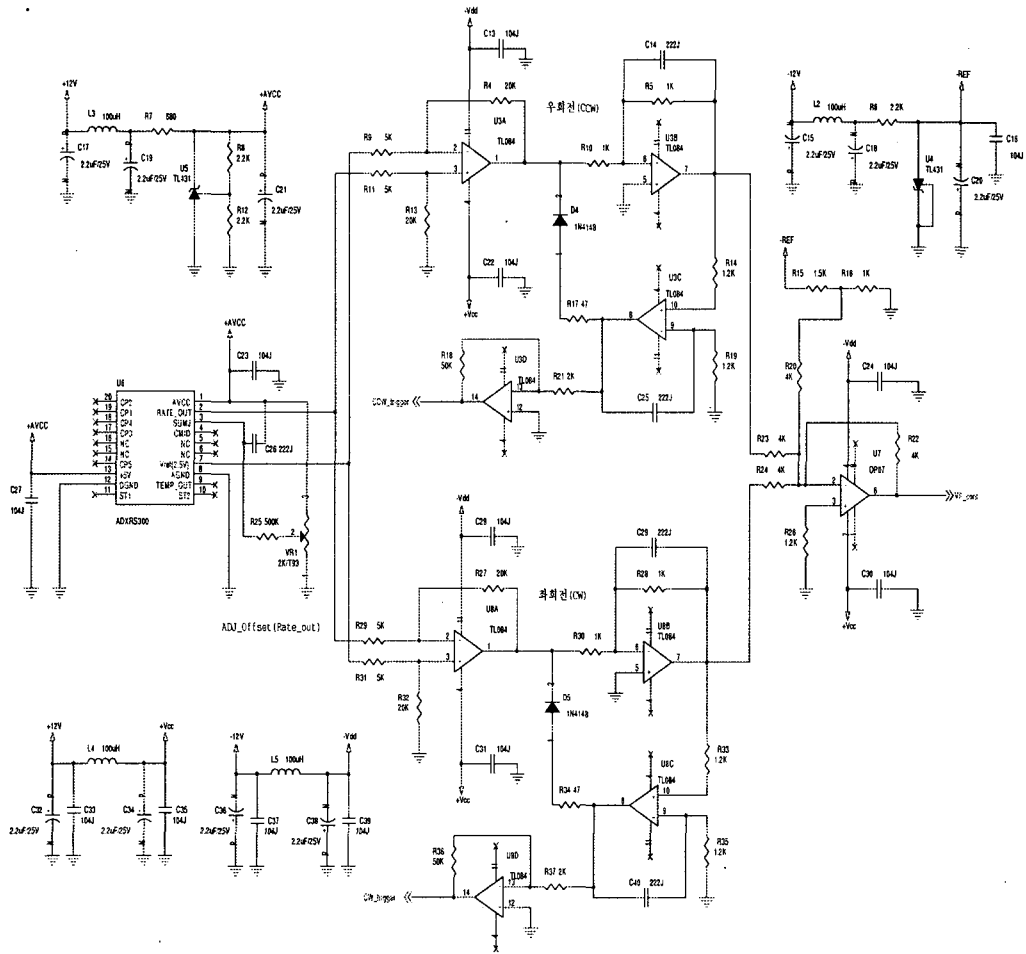
그림 3. 각속도 측정을 위한 회로도
