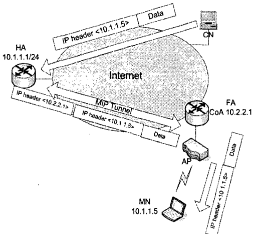
그림 1. Mobile IP Tunneling.
