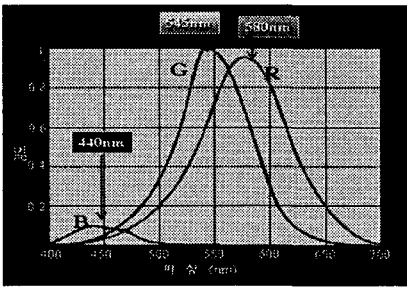
그림 1. 우리의 망막에 있는 추상체가 인지하는 파장별 자극의 정도
