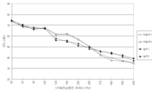
그림10. 설비 유무간 중량충격음 차단성능 비교(거실)
