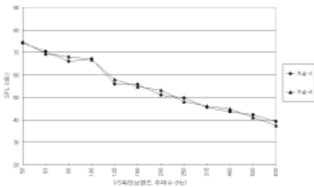
그림6. 스프링클러 설치세대의 차단성능 (거실)
