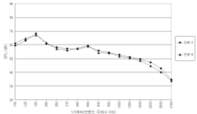
그림3. 스프링클러 설치세대의 차단성능 (안방)
