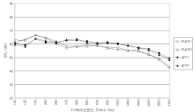
그림8. 설비 유무간 경량충격음 차단성능 비교(거실)
