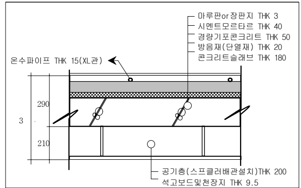
그림2. 스프링클러설비 설치 세대 단면도
