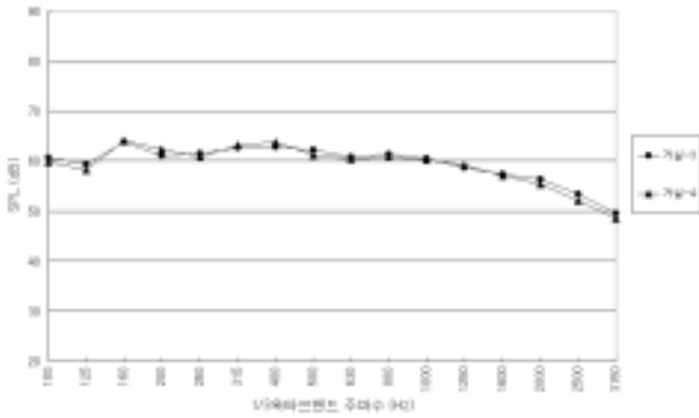
그림4. 스프링클러 설치세대의 차단성능 (거실)
