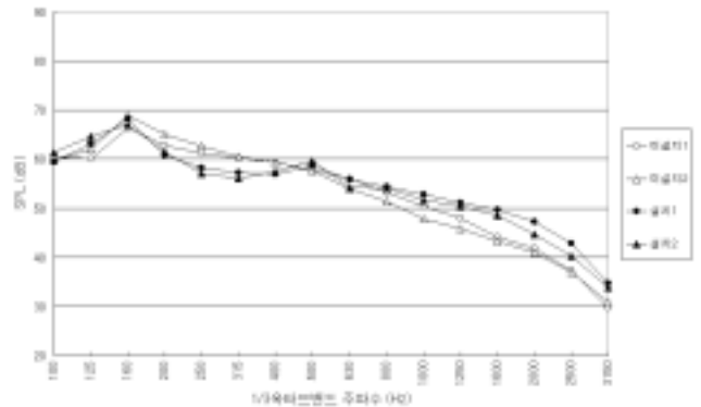
그림7. 설비 유무간 경량충격음 차단성능 비교(안방)
