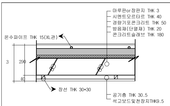
그림1. 스프링클러설비 미설치 세대 단면도
