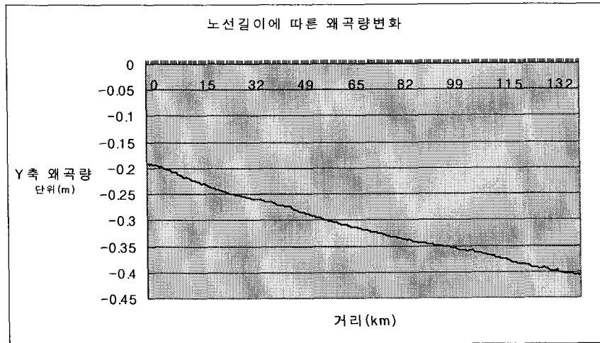
도표.5 노선길이에 따른 Y축 변위량의 변화
