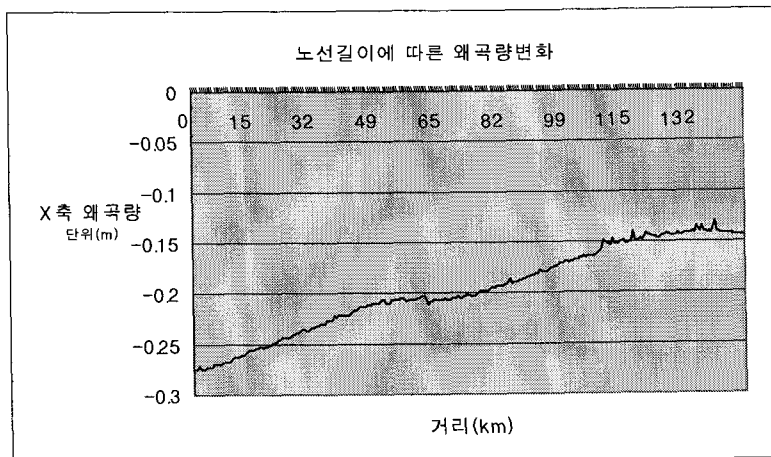
도표. 4 노선길이에 따른 X축변위량의 변화
