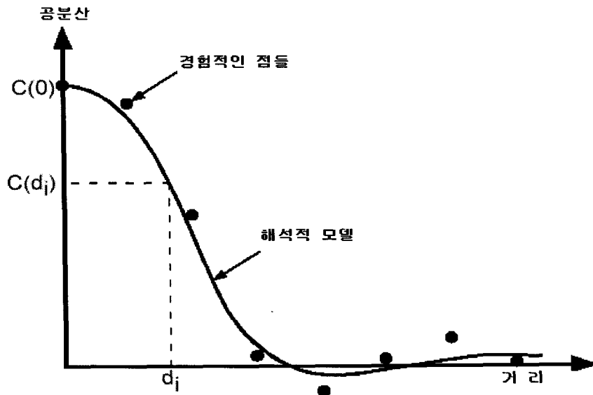
그림3. 거리에 따른 공분산함수
