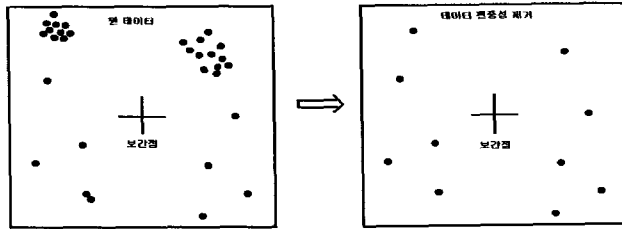
그림2. 보간과정에서 DATA Thining
