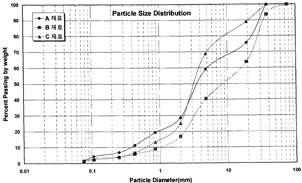
그림 3. 실험 재료별 입도분포곡선
