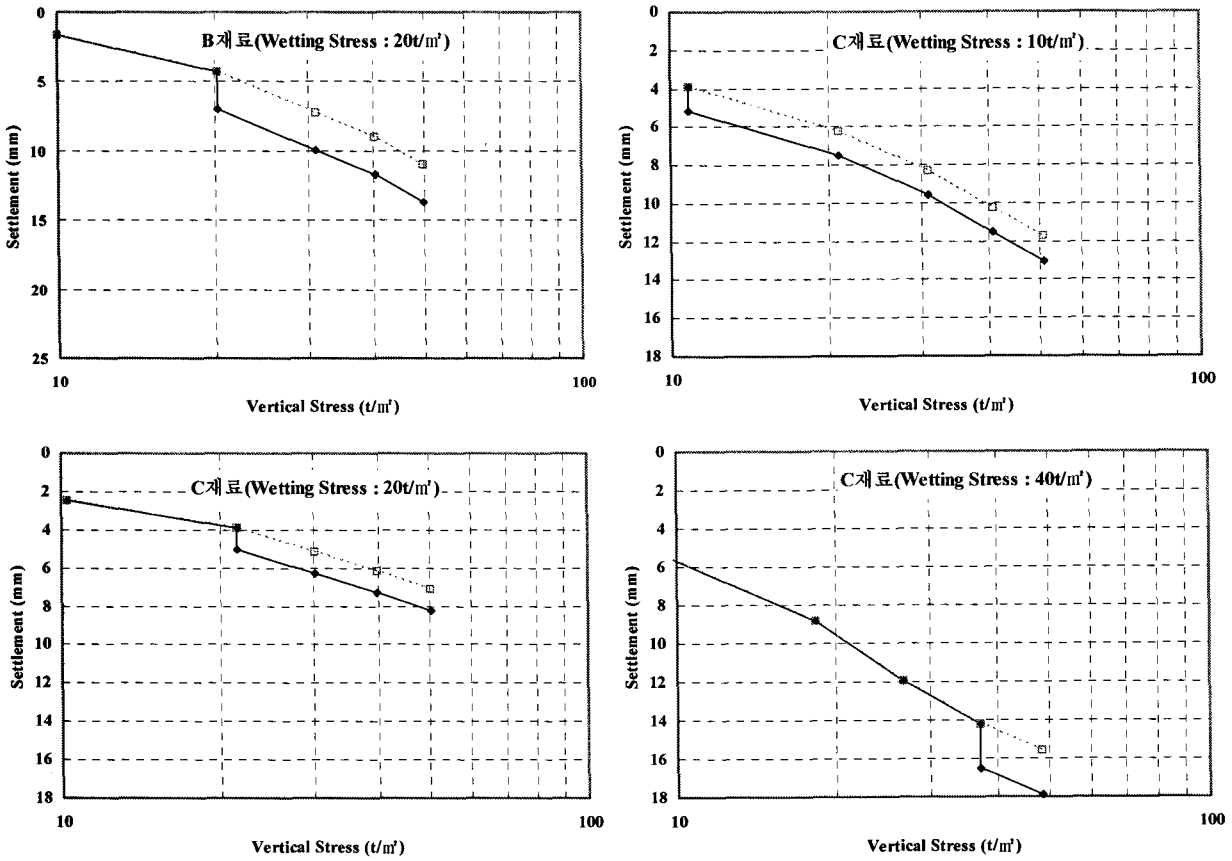
그림 7. 응력 침하곡선
