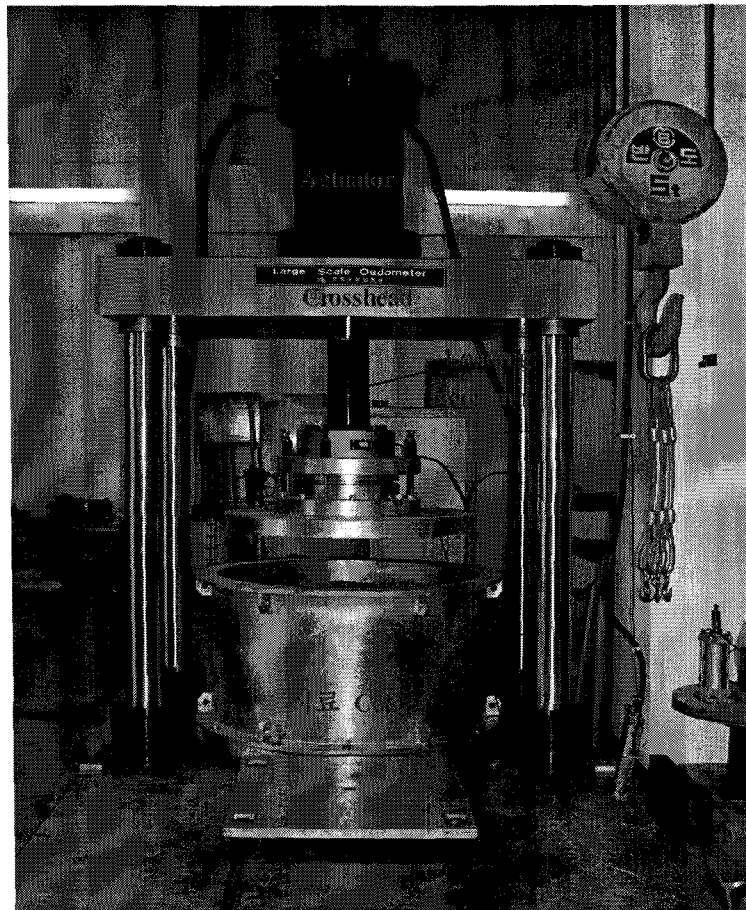
그림 4. 대형오이도미터 실험 장비 전경
