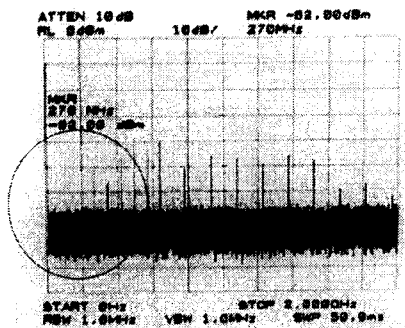
(b) 필터 통과 후 그림 8. 필터의 주파수 특성
