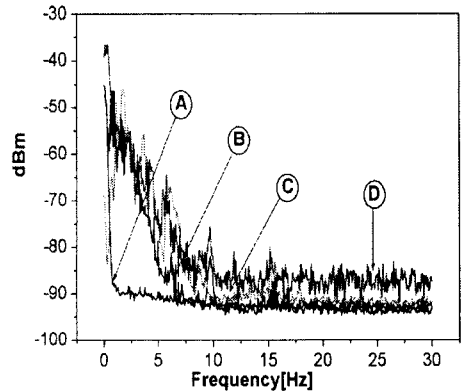
(a) 현장에서의 노이즈 주파수 스펙트럼
