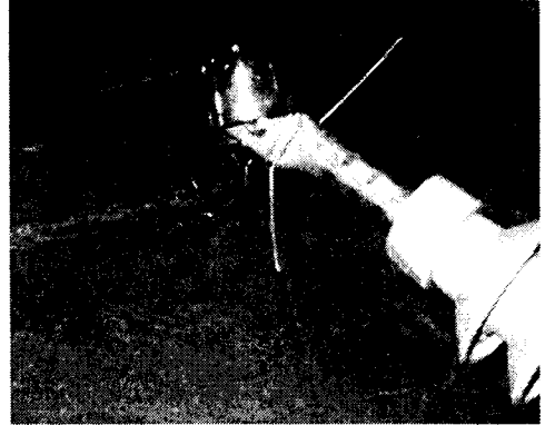
그림 5. 중단부의 모의 코로나 방전 시험
