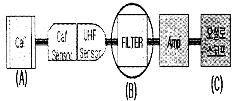
그림 6. 10~300[MHz] 까지 필터 시험 구성도
