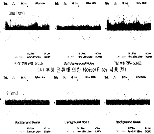
(B) Background Noise (Filter 사용 후)
