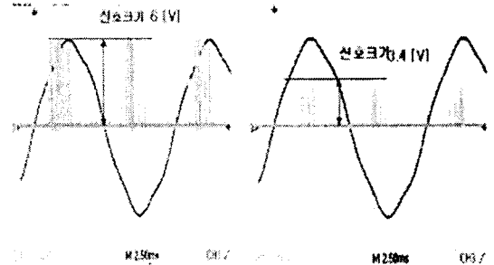
(A) 필터 없는 상태 (B) 30MHz HPF 그림 5. 모의 선로 PD 신호
