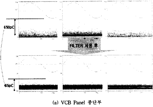
(a) VCB Panel 종단부
