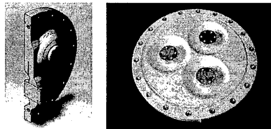
<그림 4> 센서가 내장된 스페이스 시제품
