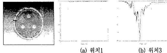
(a) 위치1 (b) 위치3 그림 7. 스페이서 위치별 반사손실(S11)
