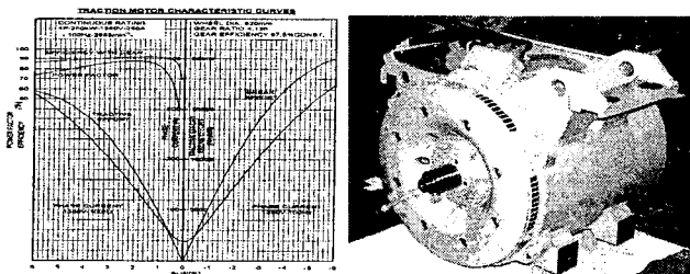
<그림 2> 견인전동기 특성곡선 및 시작품
