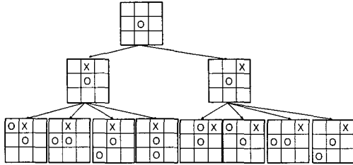
그림 3. Tic-tac-toe 문제의 트리 표현
