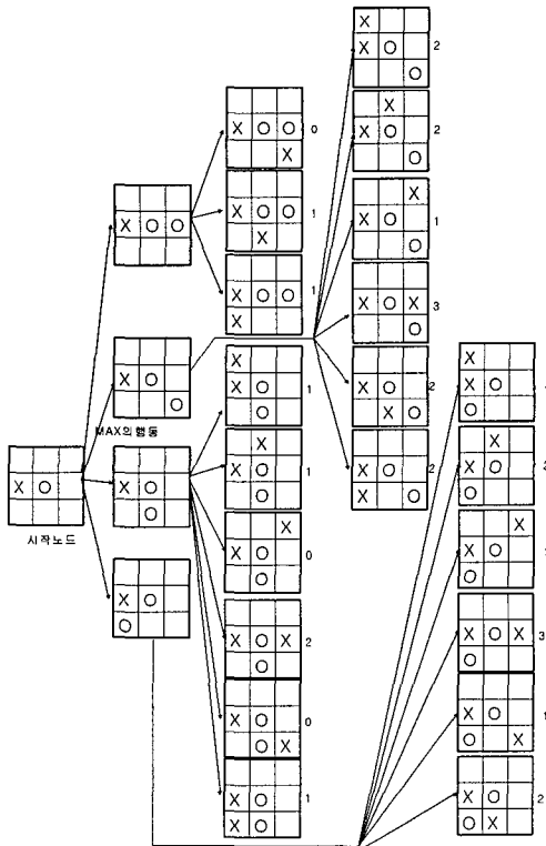
(b) 1단계 트리 탐색
