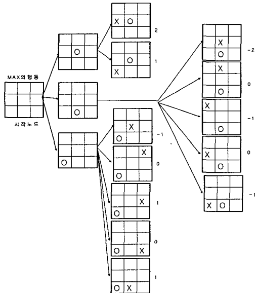
(a) 1단계 트리 탐색
