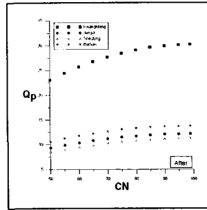
그림 10. 첨두유량-CN(개발후)
