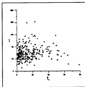
그림 5. 강우강도 -도달시간 관계비교
