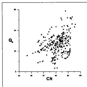
그림 7. 비유량-CN 관계비교
