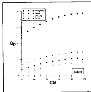
그림 9. 첨두유량-CN(개발전)
