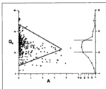
그림 6. 비유량-면적 관계비교
