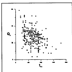
그림 3. 비유량 -임계지속시간 관계비교
