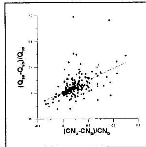
그림 8. 비유량-CN (무차원화)
