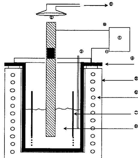
① : DC-Rectifier ② : Graphite Anode
