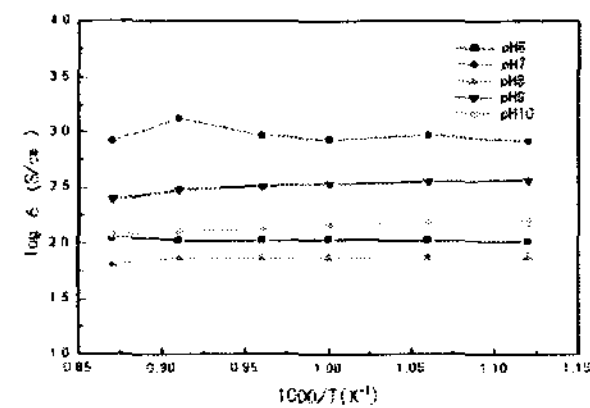
그림 4. pH 변화에 따라 합성한 LSCF의 전기전도도
