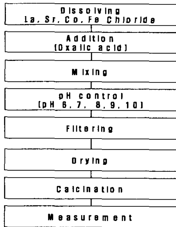
그림 1. Modified oxalate method를 이용한 LSCF 합성공정도
