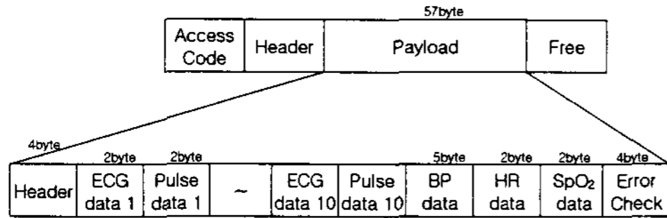
그림 5. 데이터 패킷의 페이로드 구조 Fig. 5. The structure of data packet
