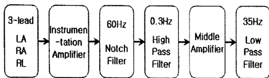
그림 3. 심전도 측정 회로 구성도 Fig. 3. The block diagram of ECG measurement circuit
