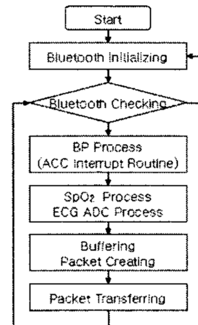
그림 4. 센서 노드 펌웨어 플로우차트 Fig. 4. The flowchart of the firmware in sensor node
