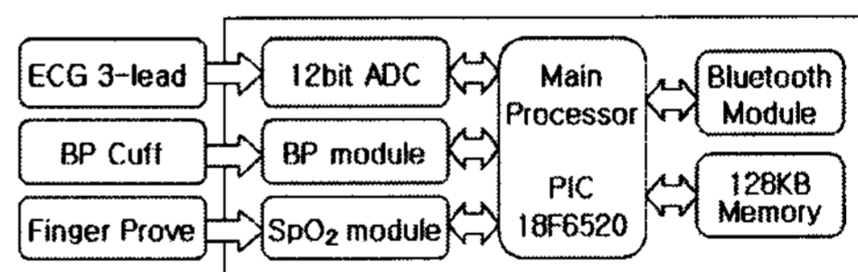
그림 2. 센서 노드 구성도 Fig. 2. The block diagram of sensor node
