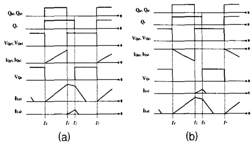
그림 2. 입력전원부의 주요 동작파형, (a)입력전압 정방향, (b)입력전압 부방향
