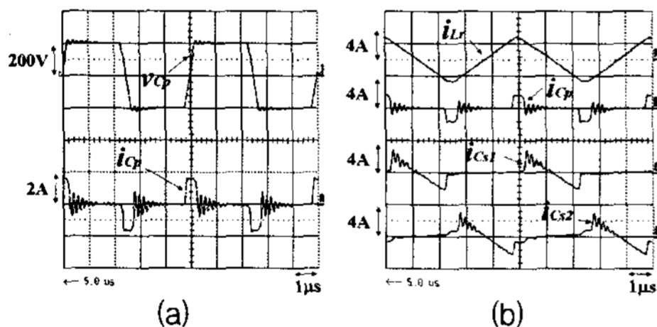
그림 5. 방전 전, (a)패널전압/전류, (b)인덕터/패널/콘덴서 전류
