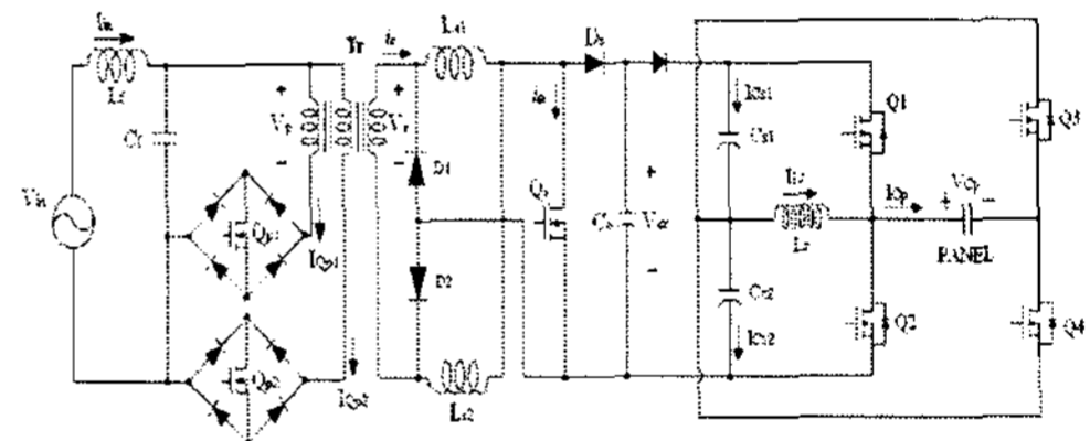
그림 1. PDP 입력전원장치와 Sustain 회로의 통합구성
