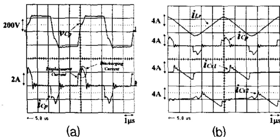
그림 6. 방전 후, (a)패널전압/전류, (b)인덕터/패널/콘덴서 전류
