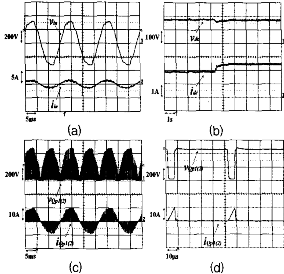
그림 4. 전압/전류 측정파형, (a)입력전압/전류, (b)부하변동에 따른 출력전압/전류, (c)입력스위치 양단전압/전류, (d)스위치 전압/전류 확대
