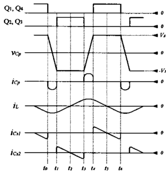
그림 3. Sustain 구동회로의 주요 파형
