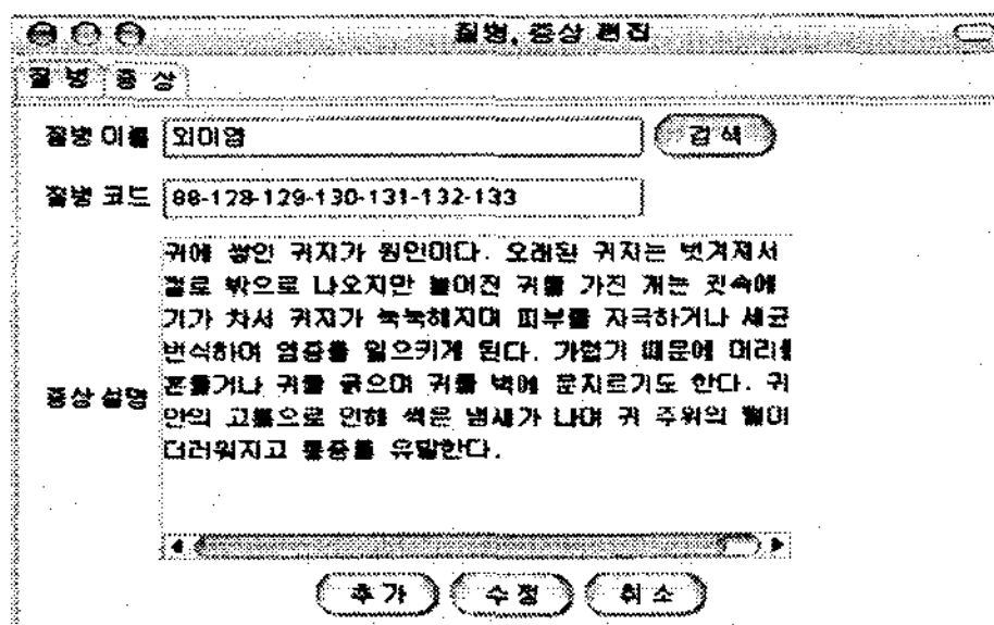
그림 4. 데이터베이스 갱신
