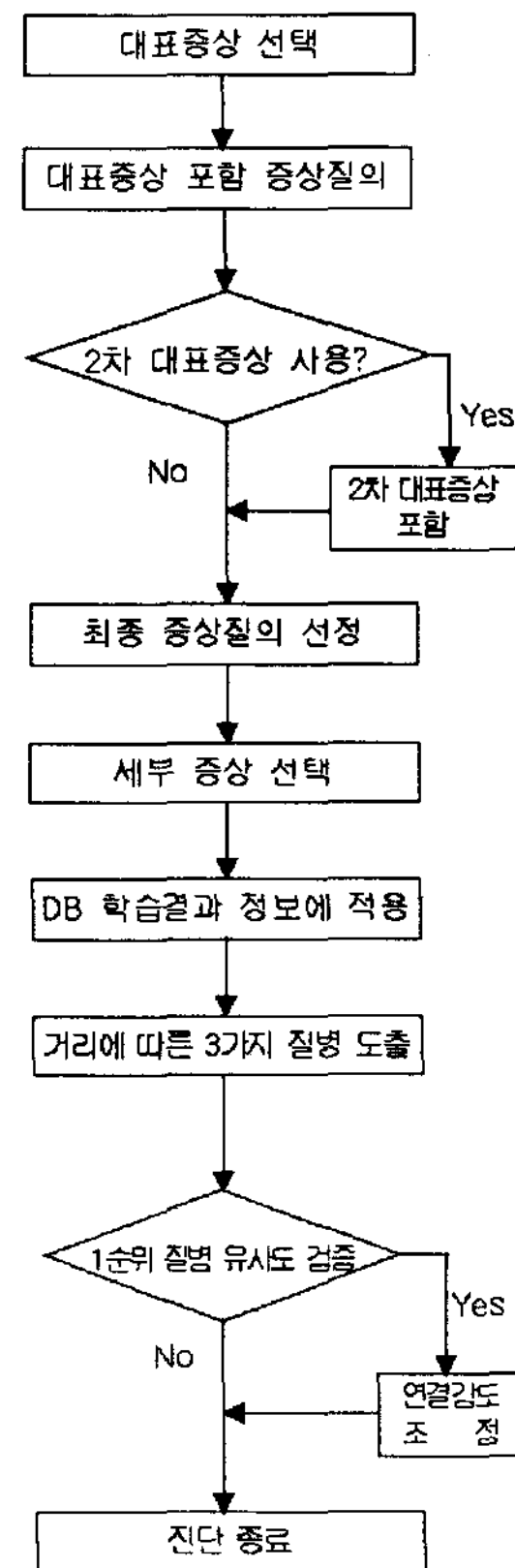
그림 5. 제안된 애견 진단 시스템
