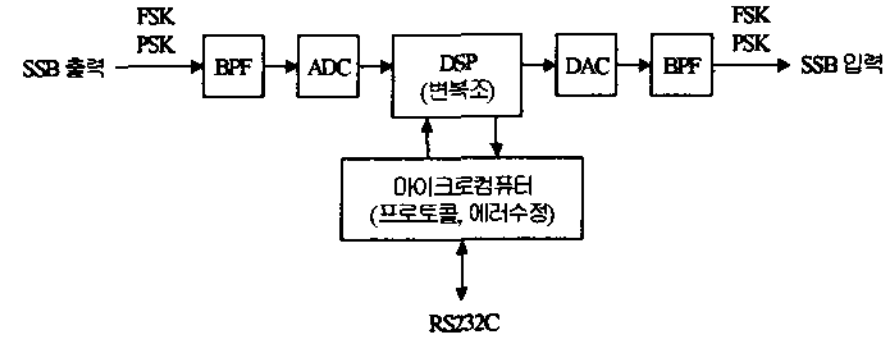
그림1. SSB 모뎀의 구성도
