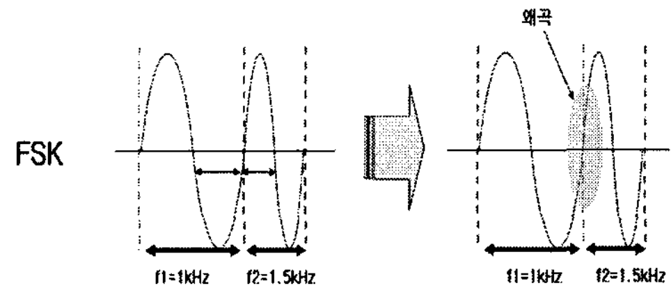
그림2. FSK 변조시 왜곡
