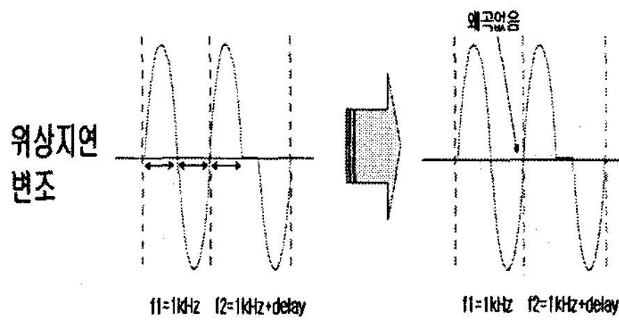
그림4. 위상지연변조 특성
