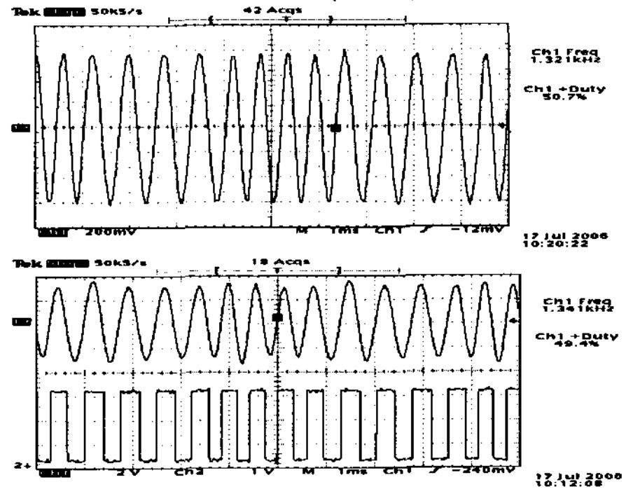
그림9. FSK 300[bps] 변·복조 파형
