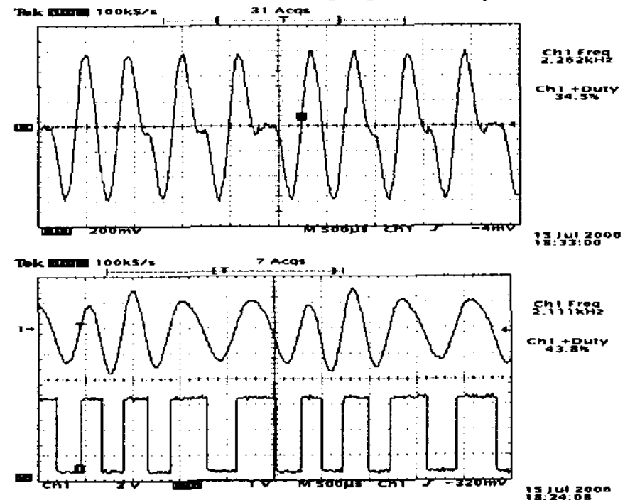
그림10. 위상지연변조 3600[bps] 파형
