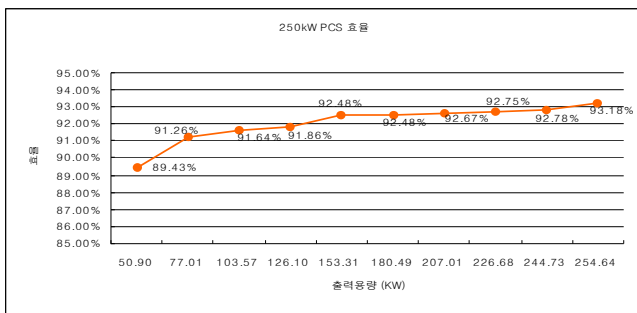
그림 7. 250kW PCS의 전부하 효율곡선 Fig 7. Efficiency curve of 250kW PCS
