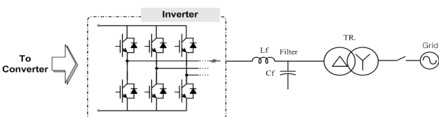
그림 4. DC-AC 인버터, 저주파변압기, 계통배전반.
