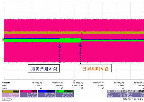
(b) 독립운전에서 연계운전으로 전환 (b). Stand-alone to Grid-connected mode
