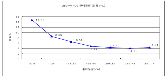
그림 8. 250kW PCS의 전력품질곡선(전류THD) Fig 8. Power quality of 250kW PCS (Current THD)
