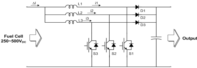
그림 2. Interleaved DC-DC 부스트 컨버터 Fig 2. Interleaved Boost DC-DC Converter
