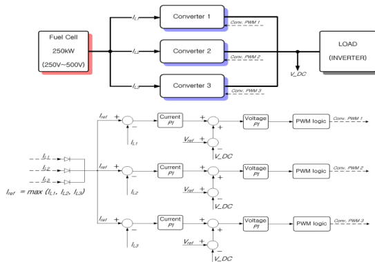
그림 3. DC-DC 컨버터 제어블럭도 Fig 3. Control block diagram of DC-DC boost converter
