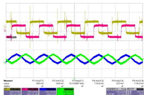
(a) DC-DC 컨버터 스위칭 및 인덕터 전류파형 (a) DC-DC converter Switching & Inductor current
