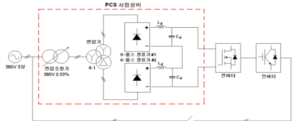
그림 5. 250kW급 PCS 시험설비 Fig 5. Test bench of 250kW PCS
