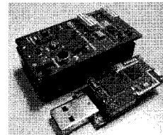
<그림 1> Kmote와 다중 센서 플랫폼
