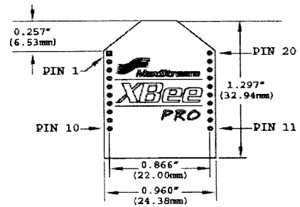
그림 1. 사용되어진 ZigBee RF 모듈의 외형도
