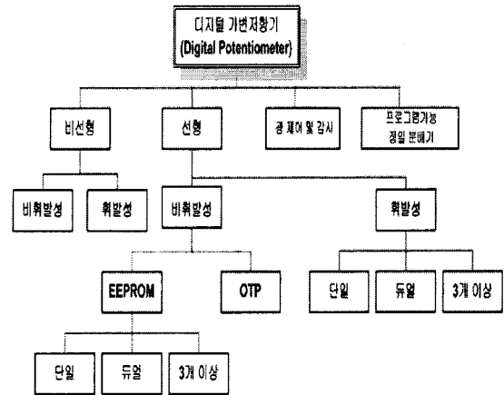
그림 5. 디지털 가변저항기의 종류
