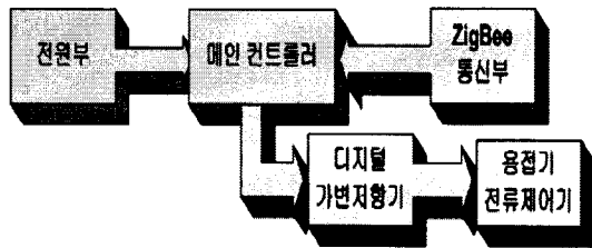
그림 3. 지그비 수신부의 회로 구성도
