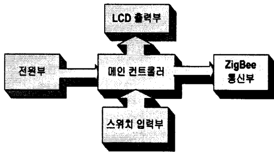
그림 2. 지그비 송신부의 회로 구성도
