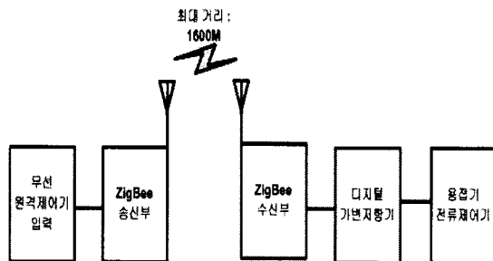
그림 4. 무선 원격제어기의 구성도
