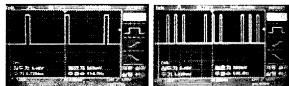
(a) 저항기의 CS 출력 (b) 저항기의 SDI 출력
