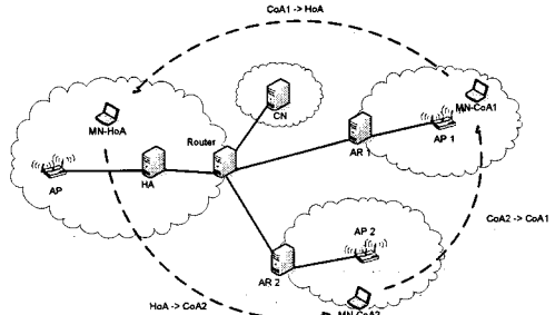
그림 1 네트워크 구성
