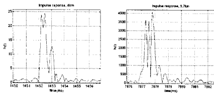
(a) 4km (b) 9.7km 그림 1. 채널 순간 응답
