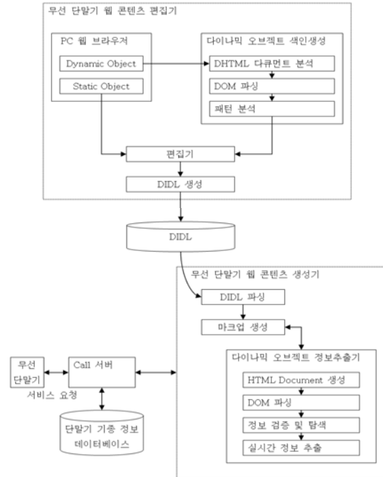
(그림 5) 다이나믹 오브젝트 서비스 구성도
