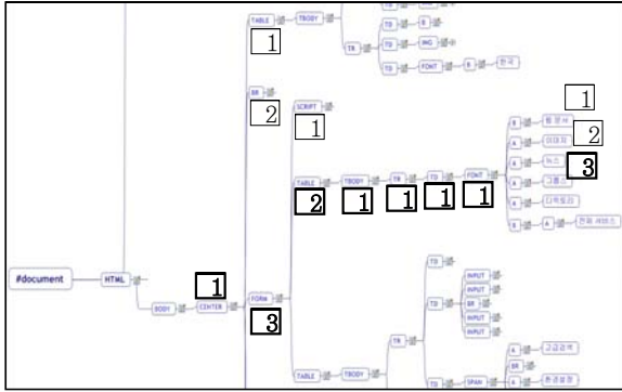
(그림 4) 구글 웹 페이지에서 “뉴스”오브젝트의 DOM구조
