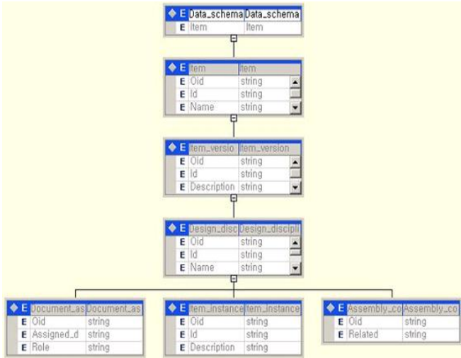
Fig. 2 XML 중립과일의 구조
