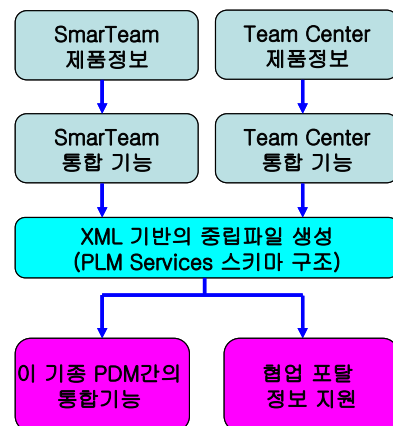
Fig. 1 상용 PDM 시스템과 협업 포탈 시스템 간의 제품 정보 교환
