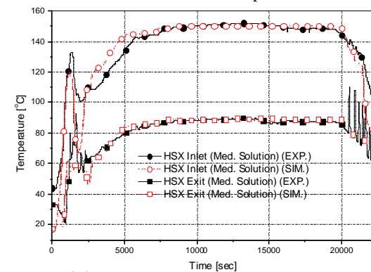
(d) HSX solution temperatures
