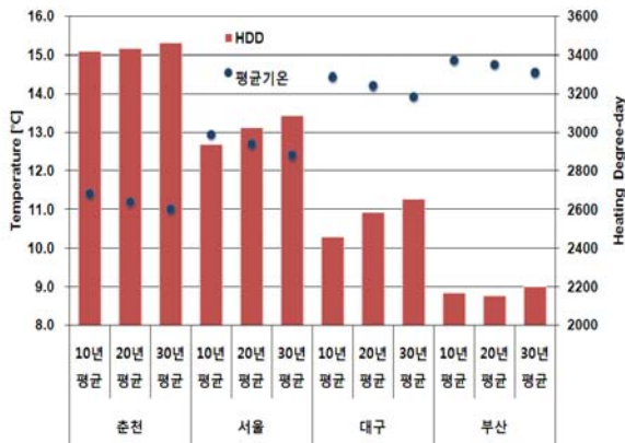
Fig. 1 주요 4개 도시의 평균기간에 따른 온도 변화와 난방도일의 변화 비교
